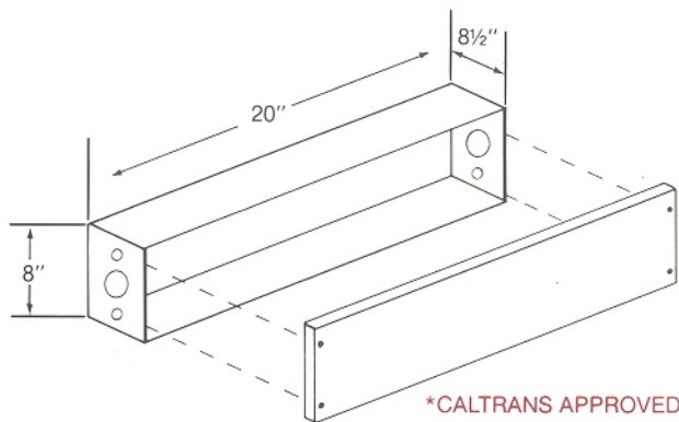
TYPE 9A PULLBOX
